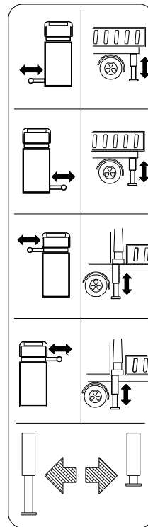
Punto morto standard Standard dead point Standardtotpunkt
